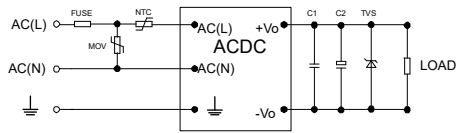
图1:AWH05-10SXX(单路)系列典型应用电路
